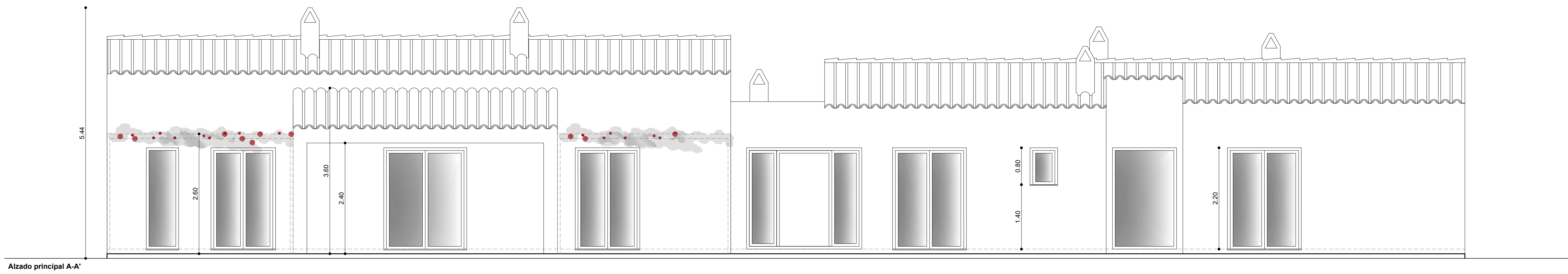
Alzado principal A-A'
